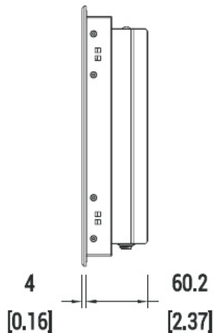
Seitenansicht
