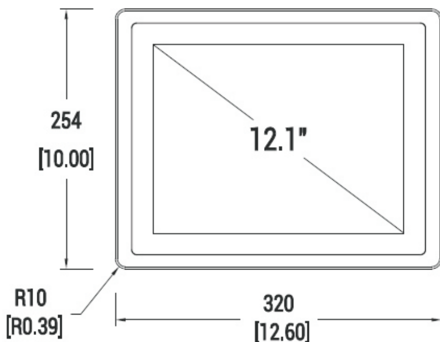
Frontansicht
