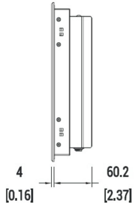
Seitenansicht
