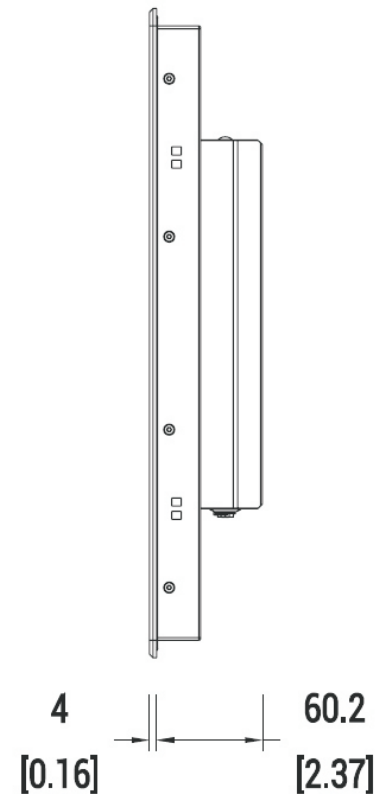
Seitenansicht
