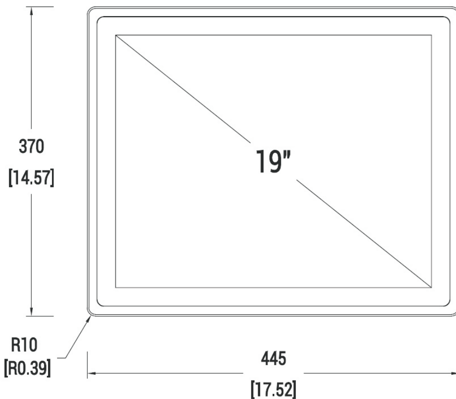
Frontansicht
